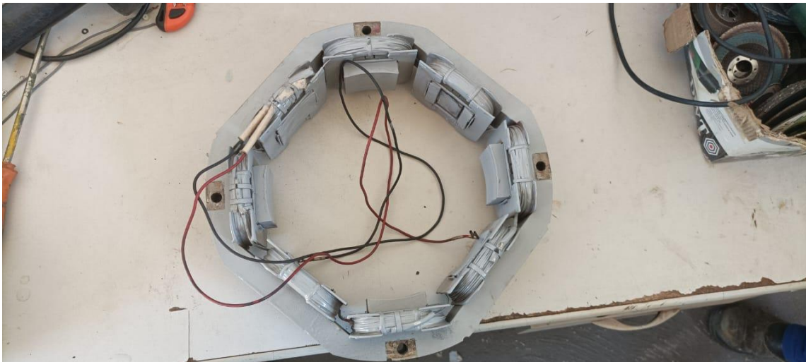
Figura 1: Excitatriz a ser rebobinada por completo.
