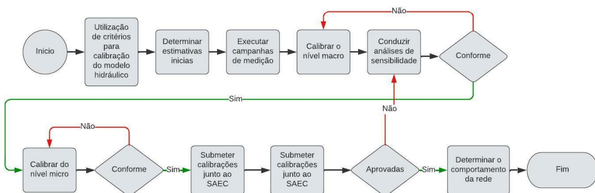
Figura 3.1. Calibração do modelo hidráulico
