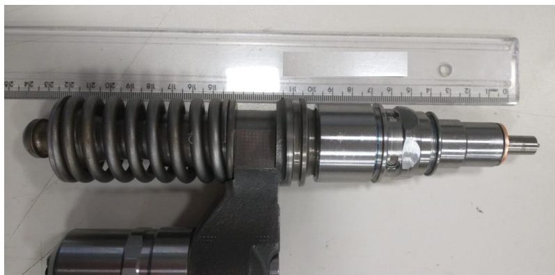
Figura 1: Exemplo de bico injetor para motor diesel DC13 072A.
