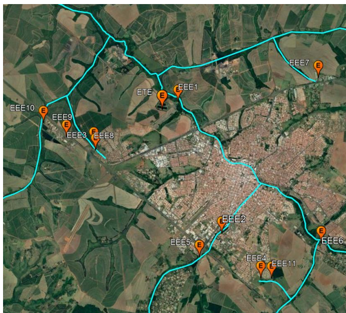
Figura 1: Localização das elevatórias de esgoto bruto e da ETE
